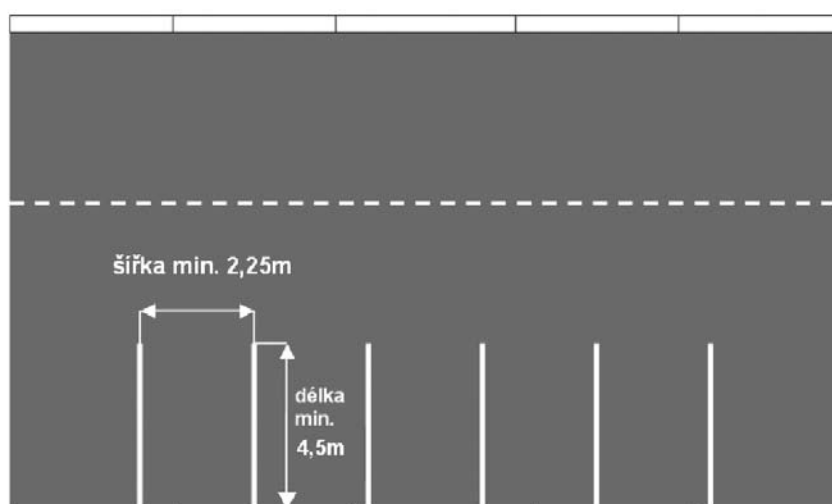
Nejmenší rozměry kolmého parkovacího místa
