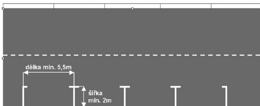
Nejmenší rozměry podélného parkovacího místa
